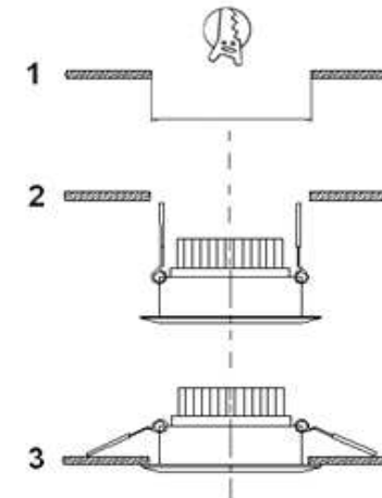
РИС. 1. Монтаж светильника
